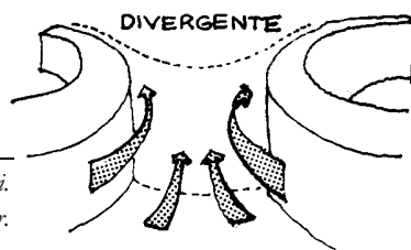
Figura 66 – Efeito de Venturi. Adaptado de Gandemer.
