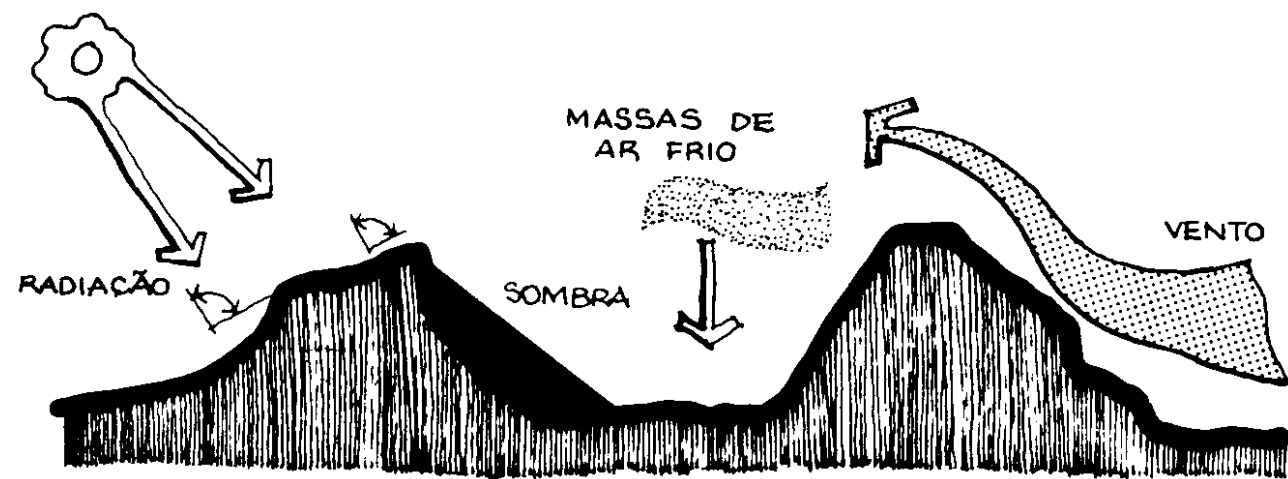
Figura 12 – Influência do relevo no microclima. Fonte: Bardou/Arzoumanian(1980).
