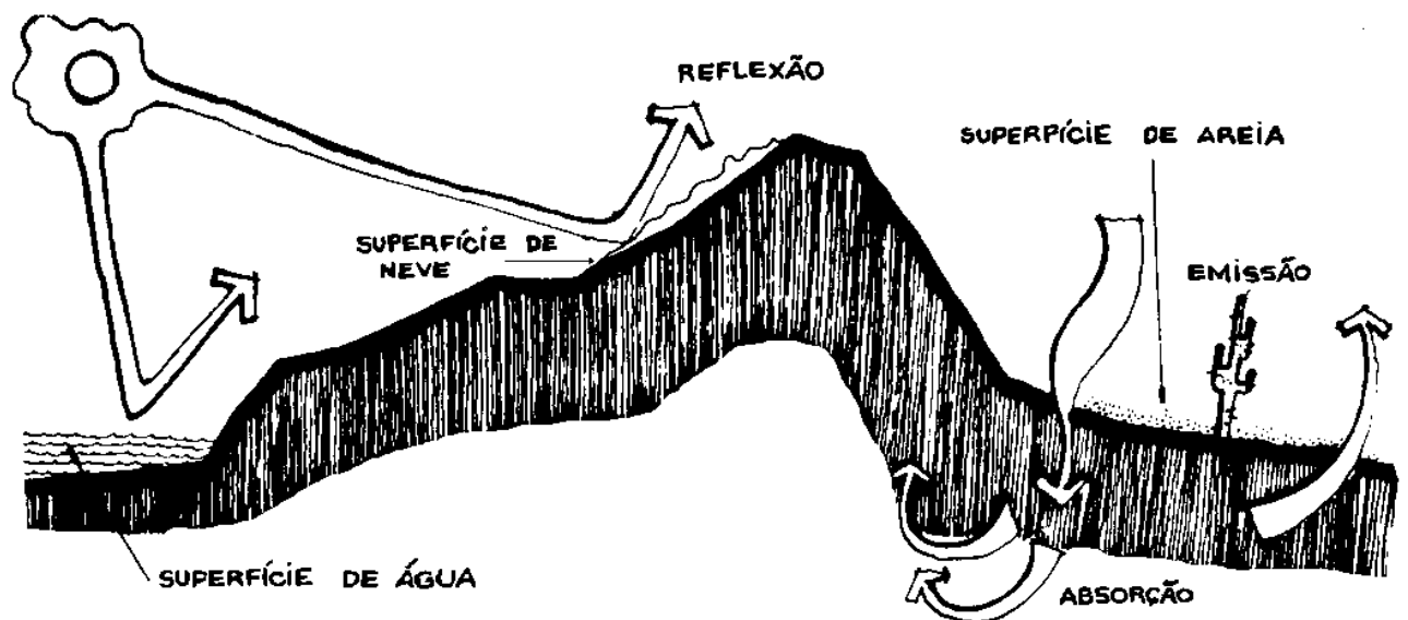
Figura 5 – Fenômenos de absorção/reflexão
