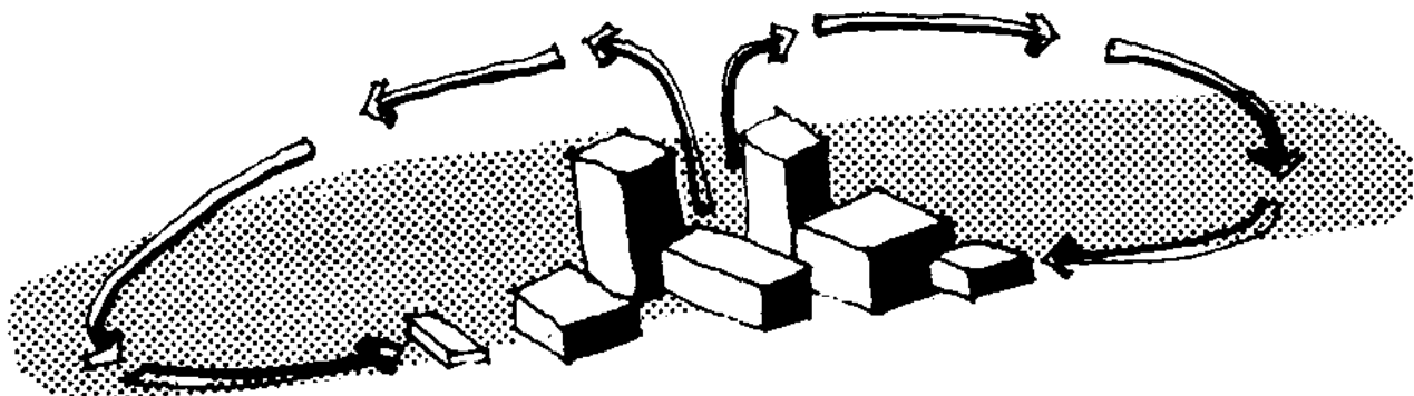
Figura 16 – Domo urbano de poeira. Adaptado de Detwyler (1974:63)..
