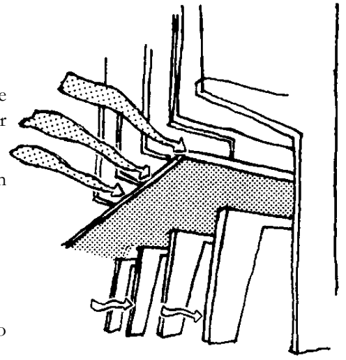
Figura 61 – Efeito de pilotis. Adaptado de Gandemer.
