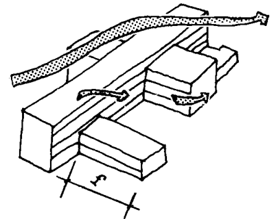
Figura 65 – Orientação a favor dos ventos dominantes. Adaptado de Gandemer.
