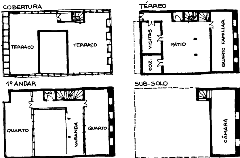
Figura 37 - Plantas de uma residência iraquiana. Fonte: "Casas orientales em Iraq" - Subbi Hussein - Al-Azzami in "Código Sociedade", Arq. Paul Oliver, (1978).
