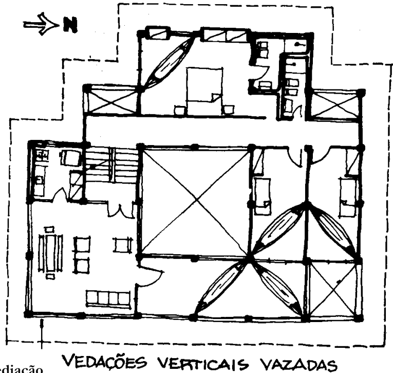
Figura 46 - Planta da residência Tarumã. Adaptado da Revista Módulo No. 53 (1979).
